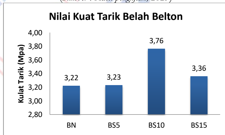
Gambar 3. Grafik nilai kuat tarik belah beton
