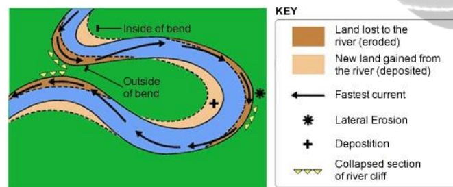
Gambar 2.2 Perubahan Bentuk Meander
