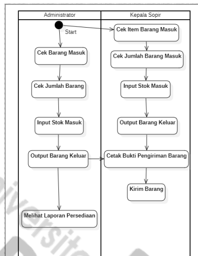
Gambar 2.2 Activity Diagram Barang Masuk dan Keluar
