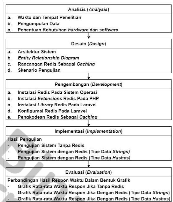
Gambar 2. Kerangka Berpikir
