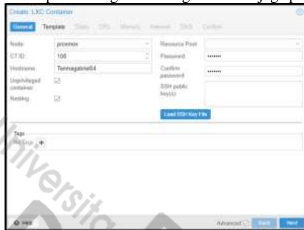
Gambar 5. Pengaturan General
