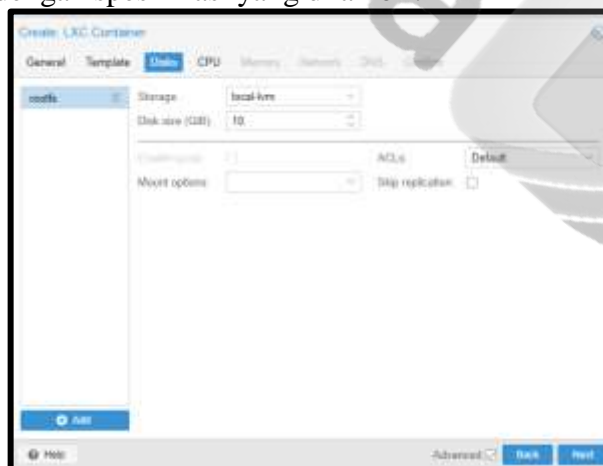
Gambar 6. Pengaturan Disks
