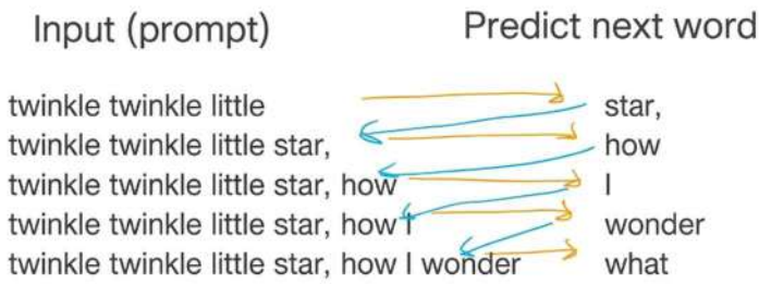
Gambar 17. Mekanisme Generatif Autoregresif melalui Prediksi Kata Berikutnya secara Berulang (Iterative Next-Word Prediction).
