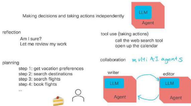
Gambar 37. Arsitektur Agen AI
