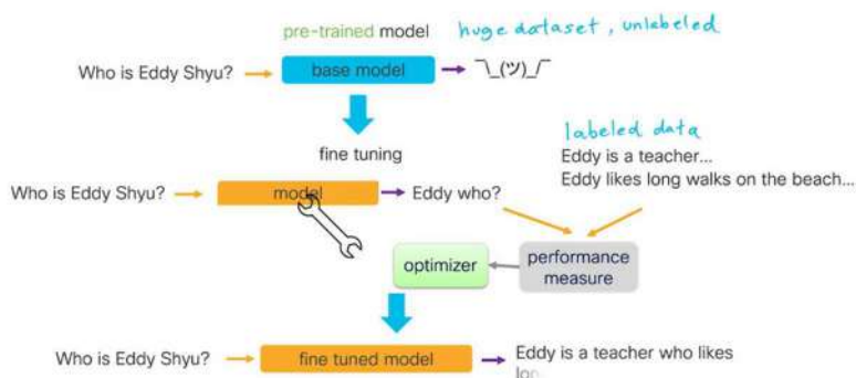
Gambar 36. Mekanisme Fine-tuning dalam Peningkatan Akurasi Model
